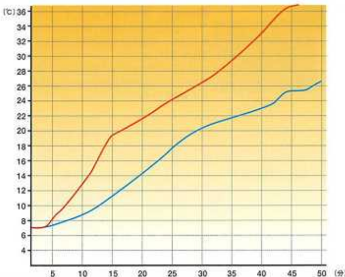
加温時室内温度推移
