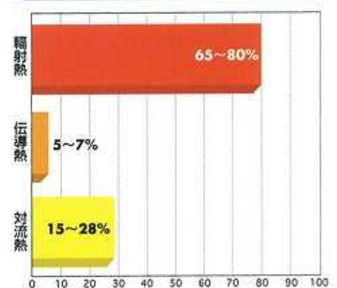
側方への熱の流れ
