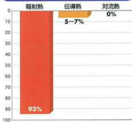
下方への熱の流れ
