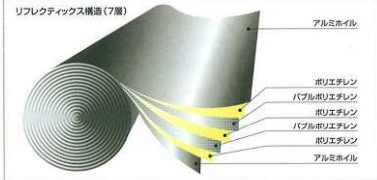
リフレクティックス構造 (7層)
